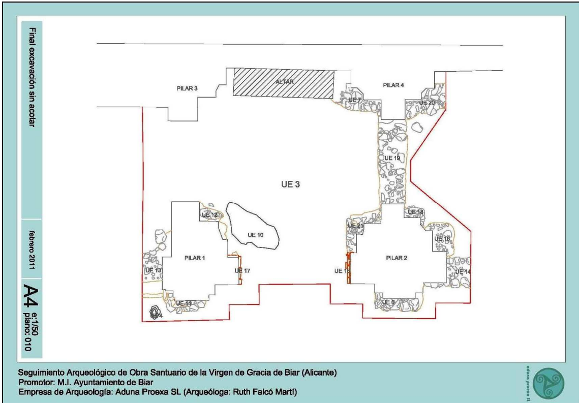
Planta de las estructuras de cimentación.
