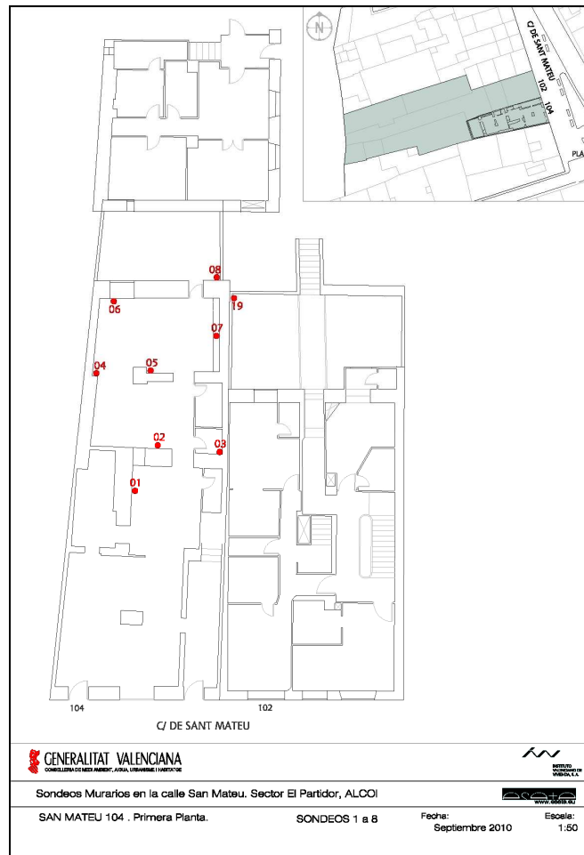
Planta general del inmueble de Sant Mateu, 104.
