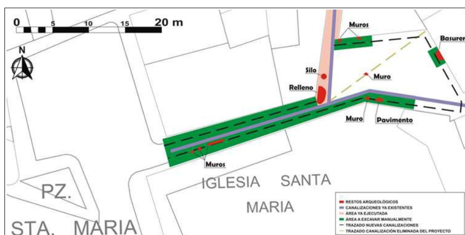
Plano de localización de la zona de excavación manual
