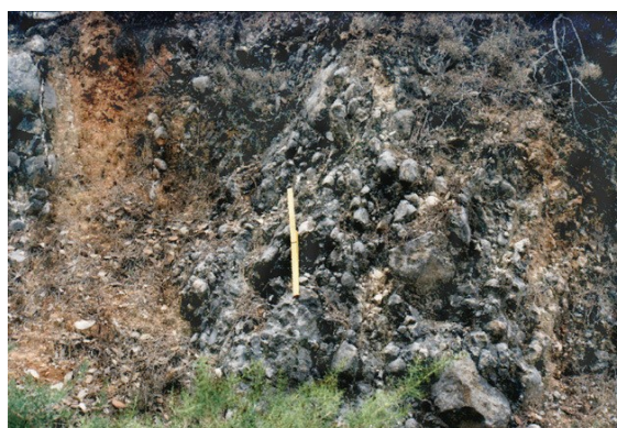
Vista del afloramiento de sílex
