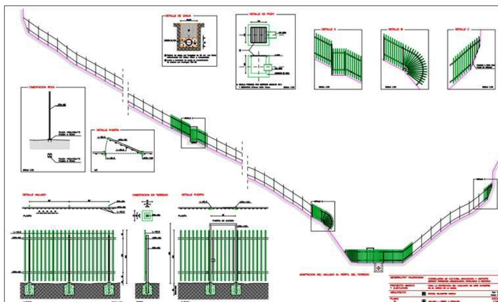
Sección y detalles del cerramiento
