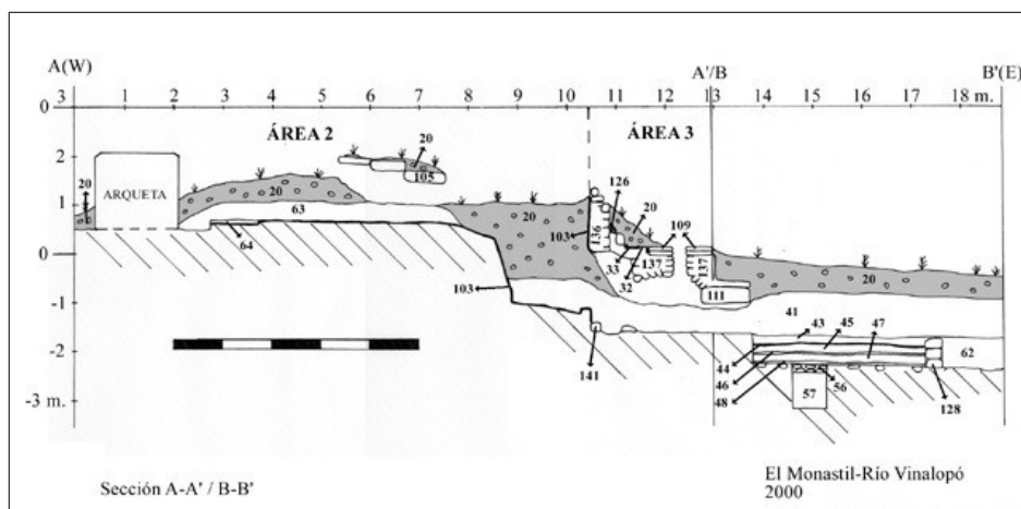
Sección A-A' y B-B'
