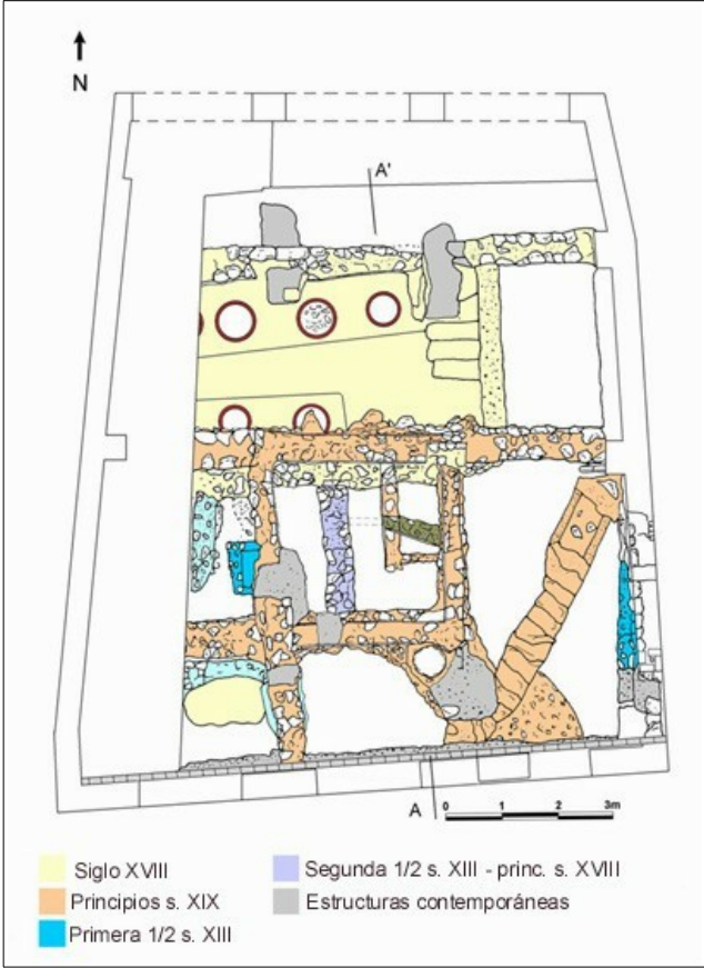
Planta general de la excavación
