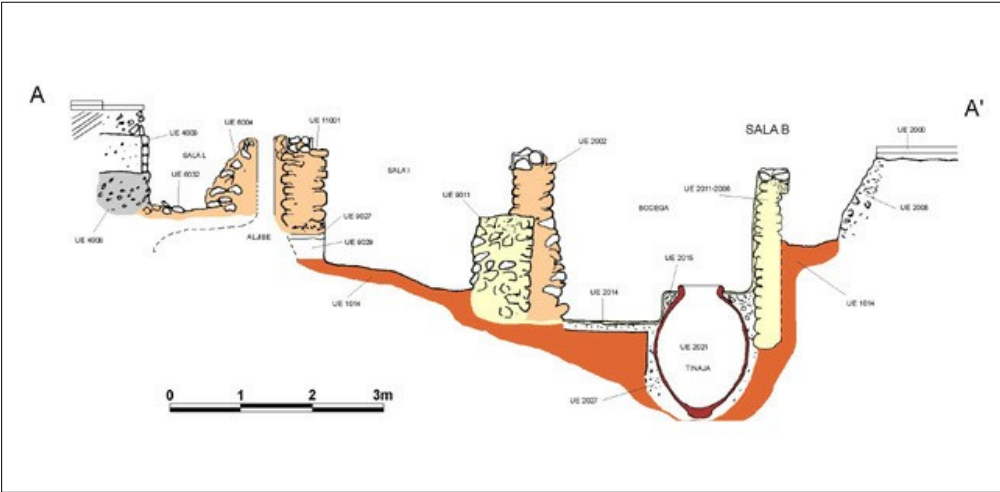
Sección transversal de la excavación. Puntos A-A'
