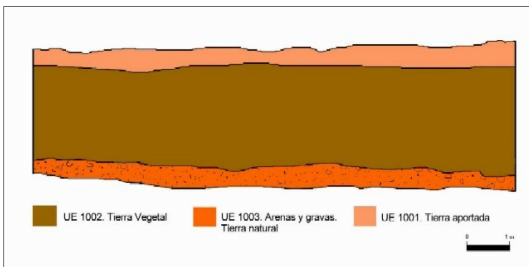
Estratigrafía del perfil sur
