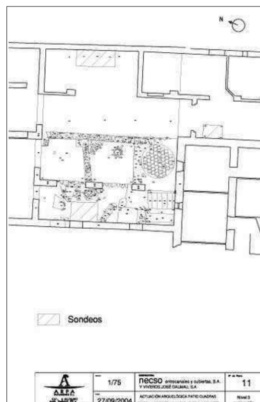
Plano excavación nivel inferior
