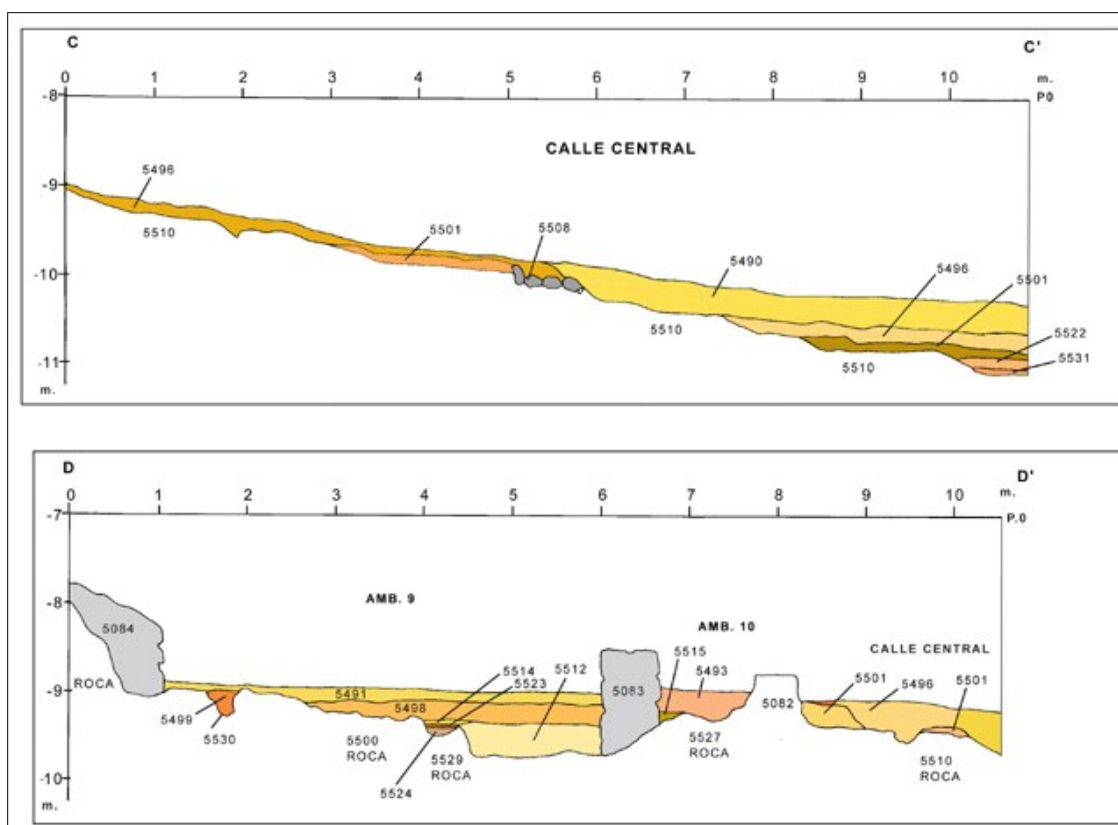
Secciones C-C' y D-D' de la campaña de 2003
