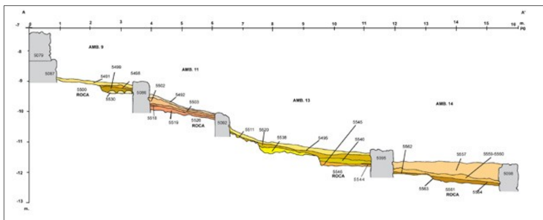
Sección A-A' de la campaña de 2003
