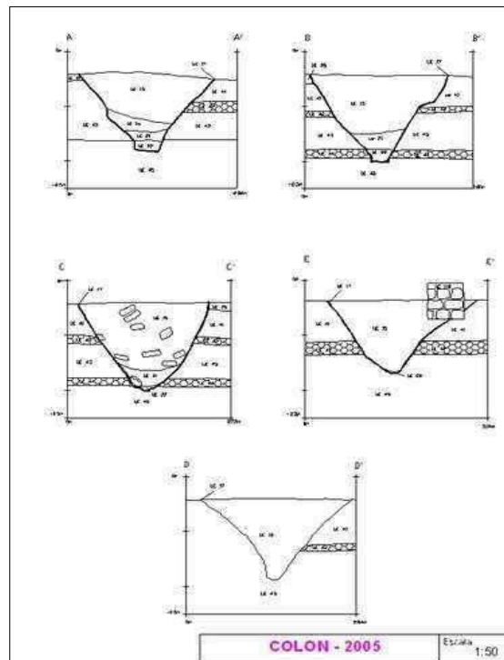
Secciones fossa fastigata
