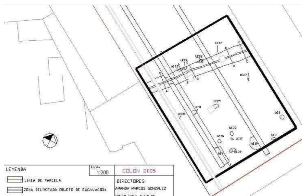
Planta general vista desde el este
