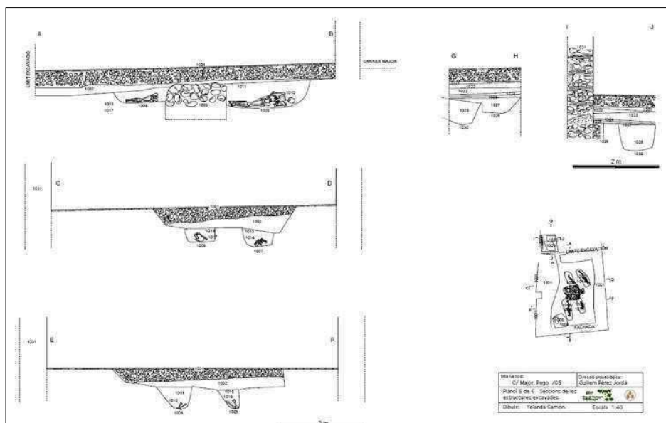
Secciones de las estructuras excavadas
