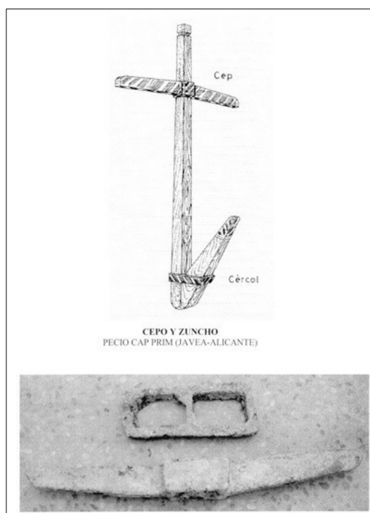
Esquema de ancla romana
