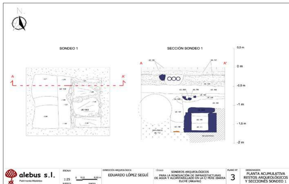
Plano de planta y secciones del sondeo 1
