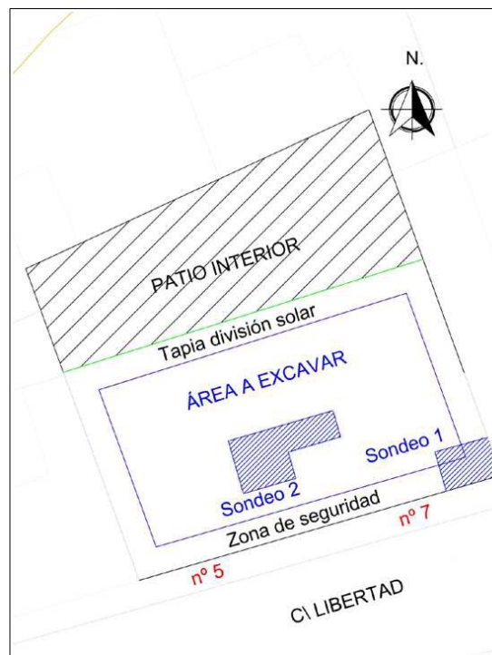
Plano con la situación de los sondeos
