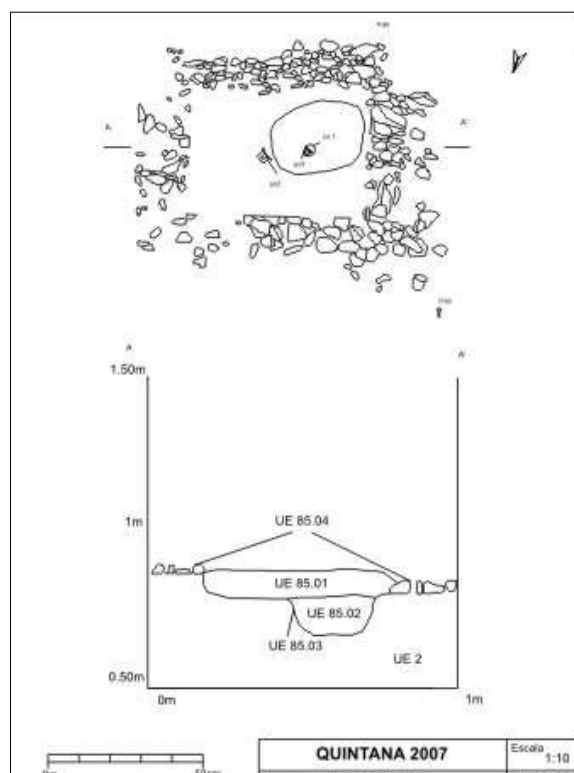
Punto 85 y 86. Planta y sección
