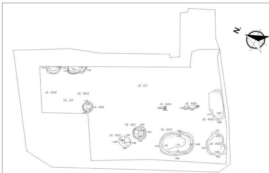
Estructuras. Fase 1
