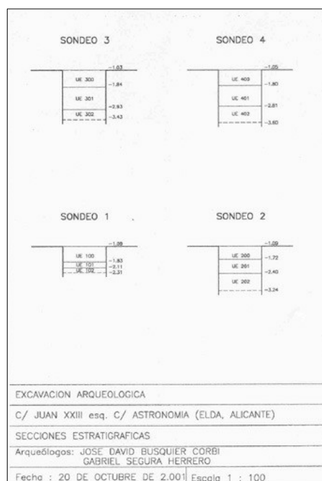
Secciones estratigráficas sondeos
