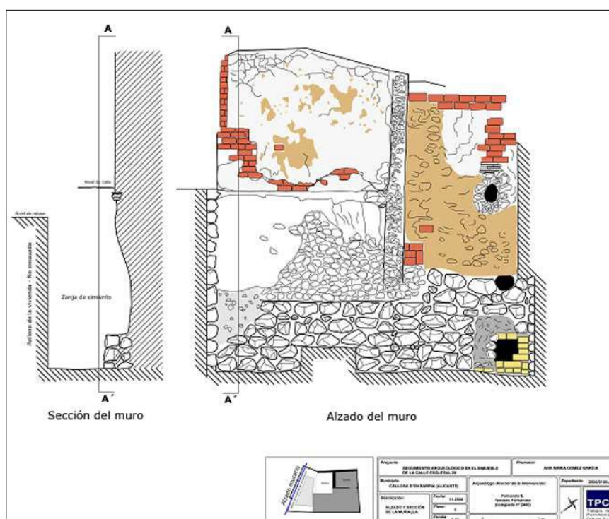
Alzado y sección de la muralla y muro del perfil E
