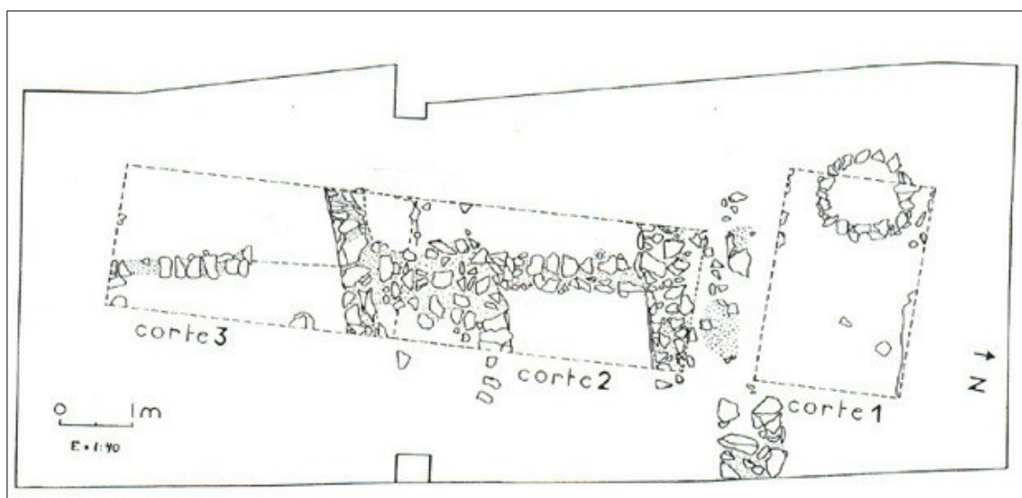
Planta general de la excavación (E/1:40)
