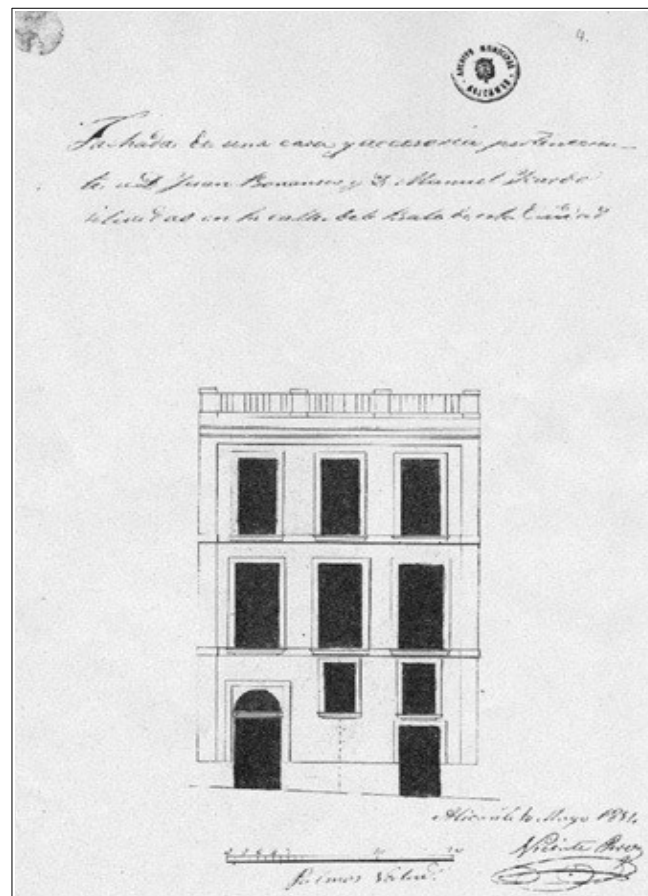
Alzado según proyecto de reedificación de 1854
