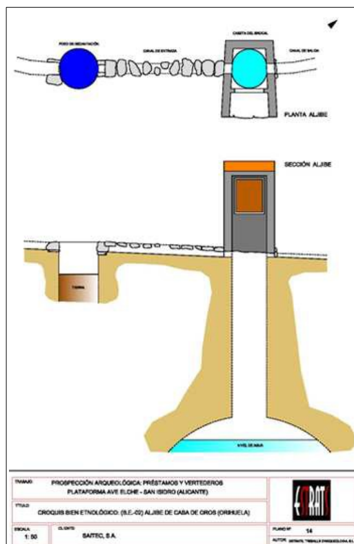
Croquis aljibe de Casa de Oros
