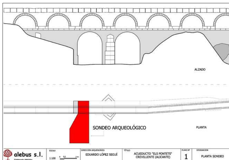
Localización del sondeo y dibujo del acueducto de Els Pontets
