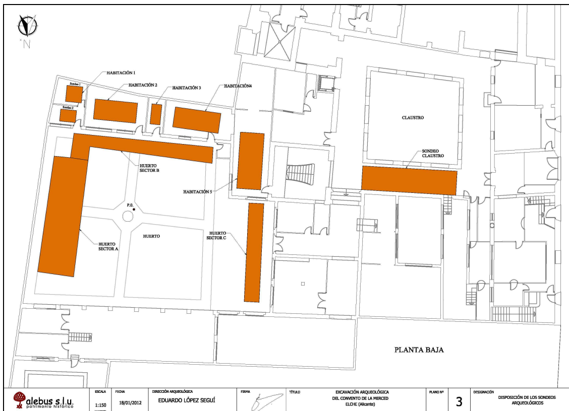
Plano de planta con distribución de los sondeos efectuados.
