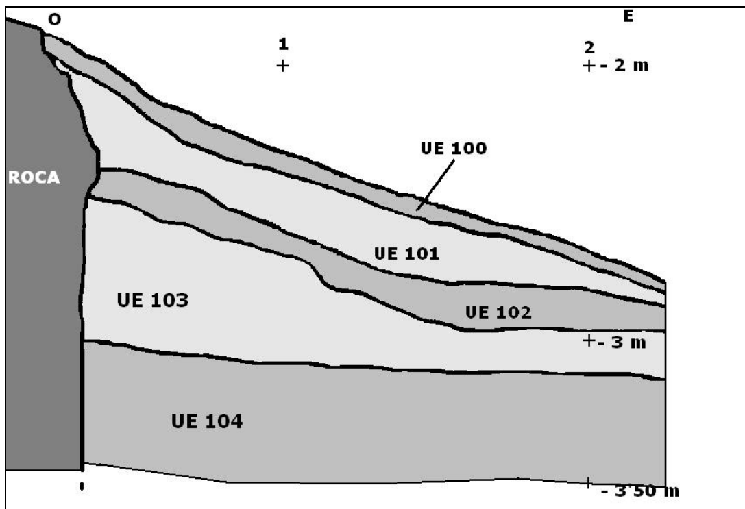
Sección A-A', con la sucesión de rellenos que colmatan la cantera.
